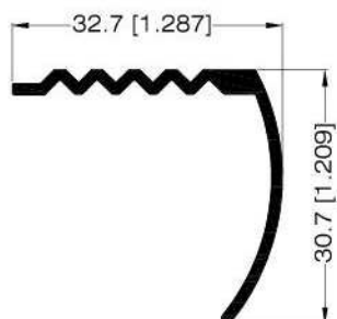
PERFIL PARA ESTRIBO 31054
