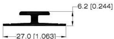
MOLDURA PARA LINOLEUM 31032
