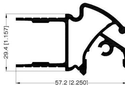
PERFIL HEMBRA BASICO 31612
