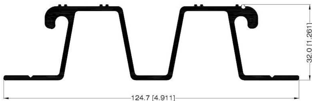
PERFIL PARA PISO 32774
