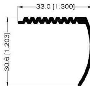
PERFIL PARA ESTRIBO 30793
