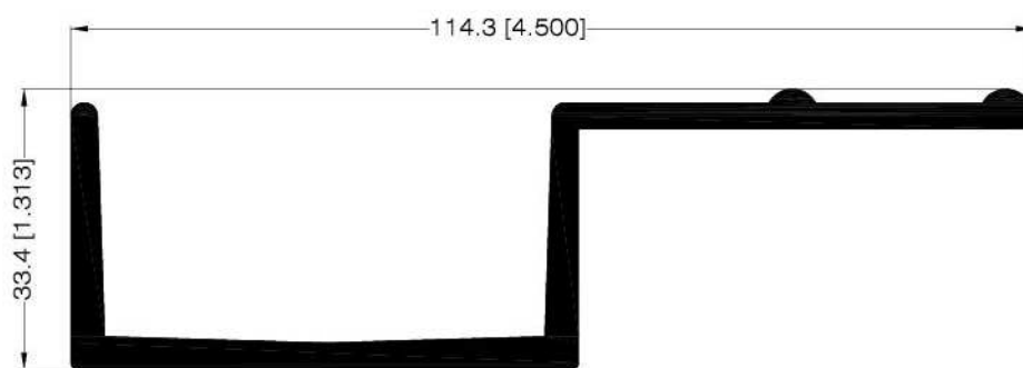
PERFIL BORDA DE 4.500\" X 1.313\" 30169
