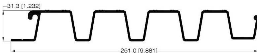
PERFIL PARA PISO 32772
