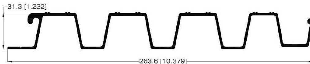
PERFIL PARA PISO 32773
