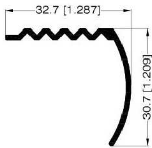
PERFIL PARA ESTRIBO 30997
